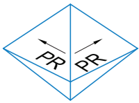
PANNEAU "PR" # 41621 4'X4' (1219mm x 1219mm) DE 0" À 2" (0 à 50mm)
