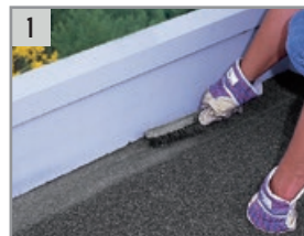
1 Remover la hojuela suelta de las membranas existentes con un cepillo metálico.
